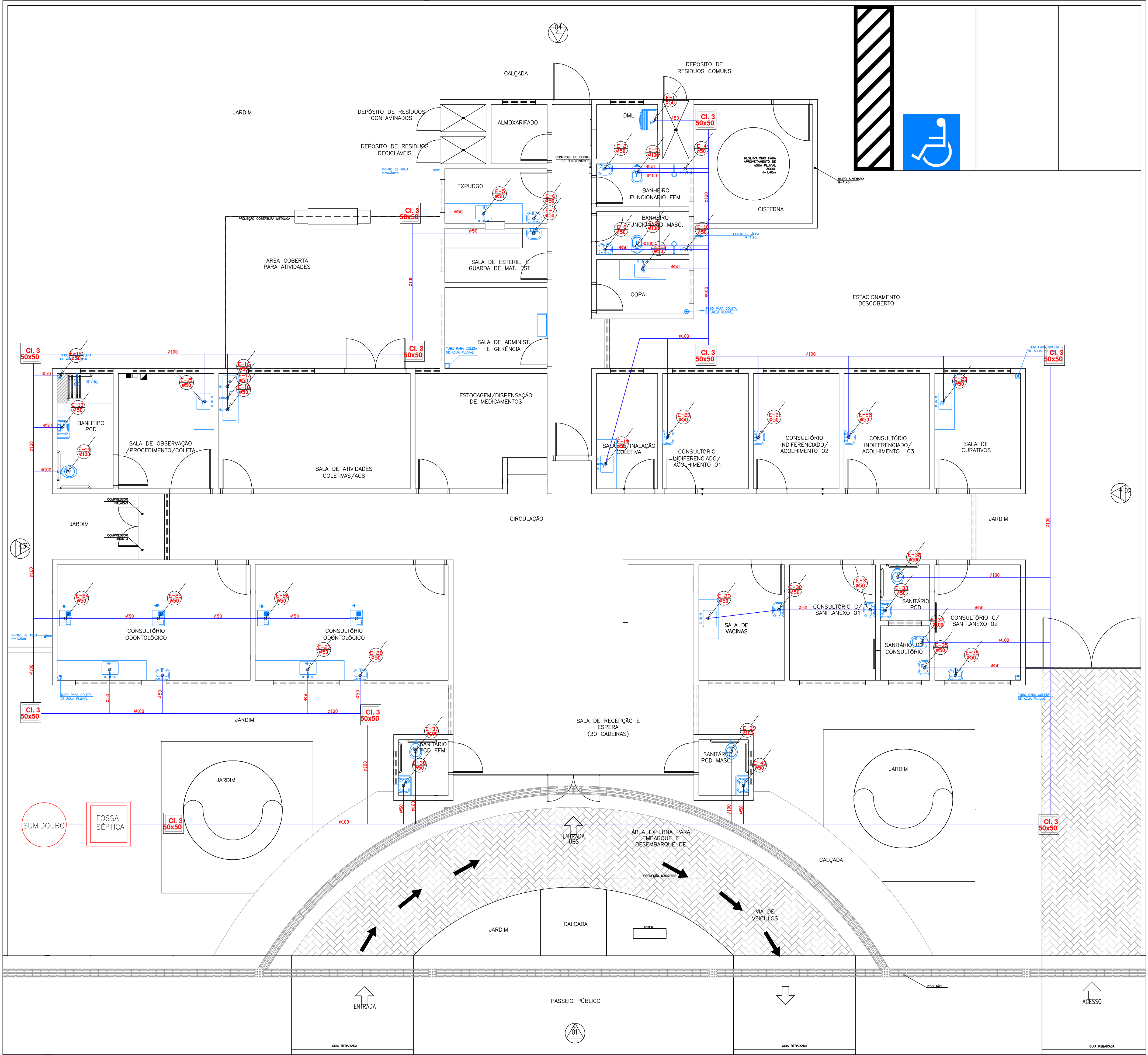
PLANTA BAIXA SANITÁRIO
