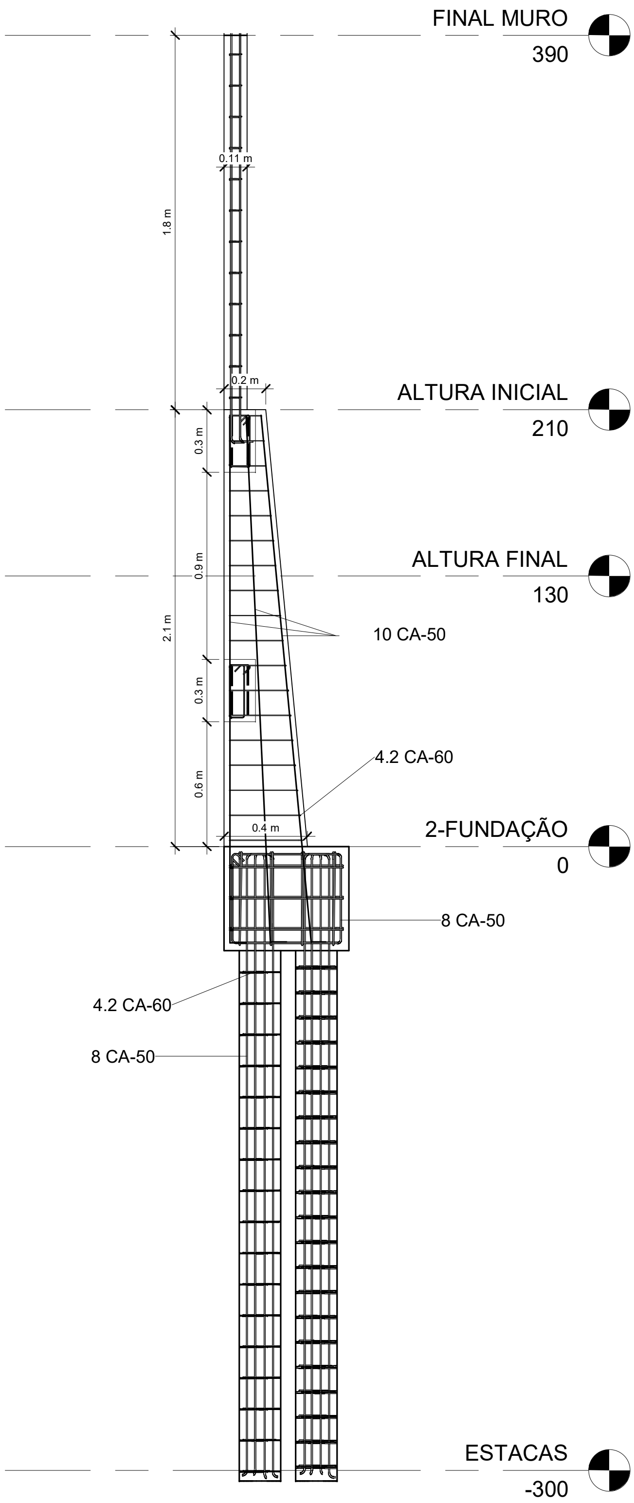
Vista Lateral Arrimo
