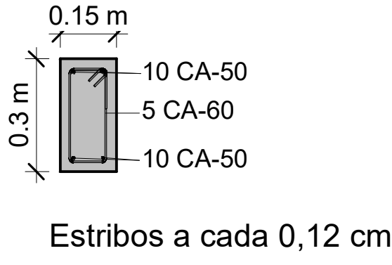
Detalhe das Vigas Arrimo
