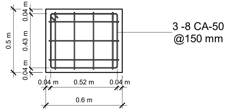
Detalhamento dos Blocos
