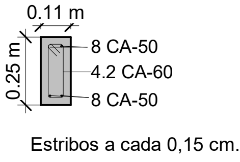
Detalhe das Colunas do muro
