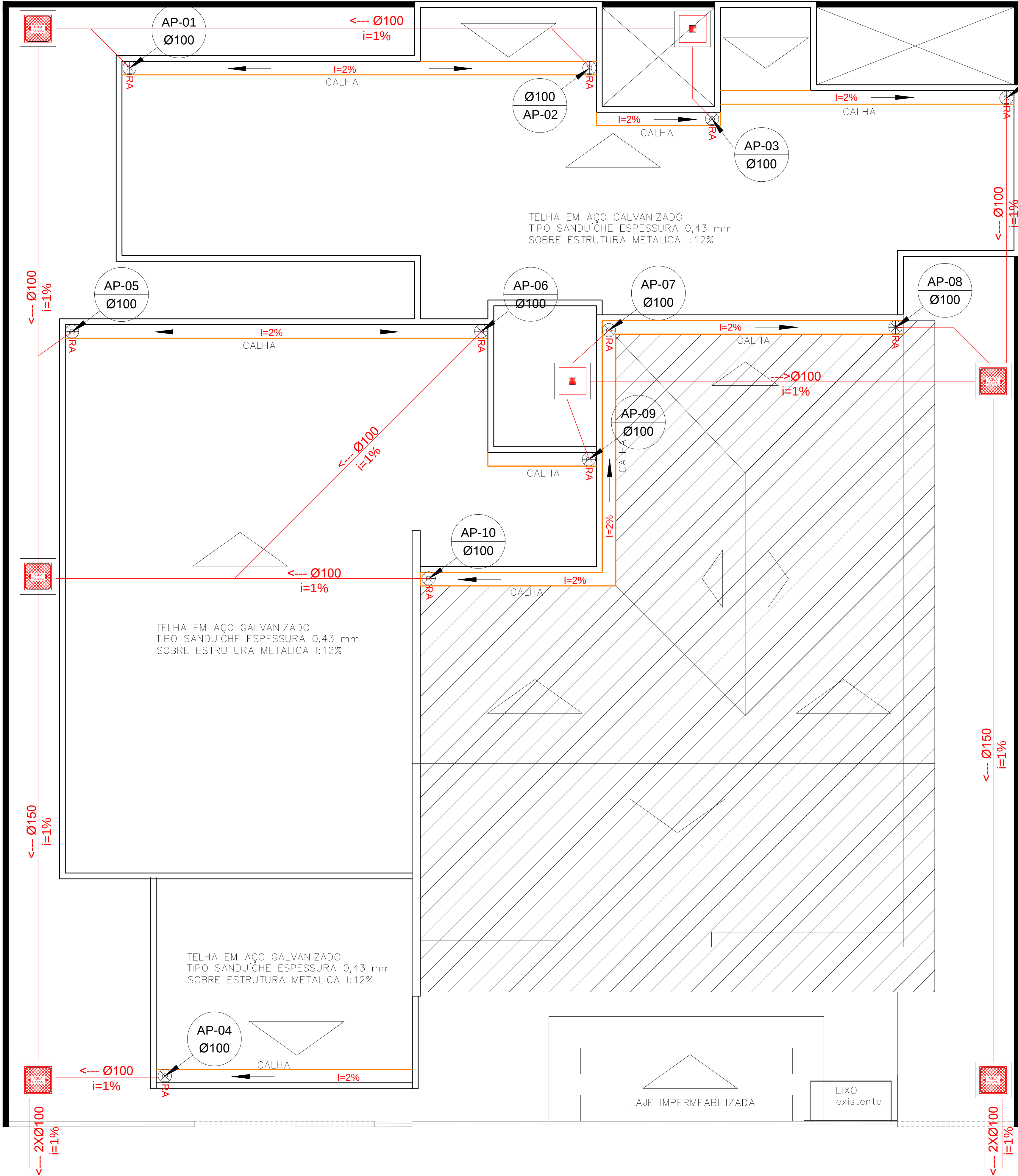
PLANTA DE COBERTURA Escala 1/50
