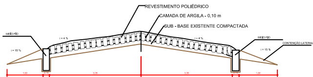
SEÇÃO TIPO PAVIMENTAÇÃO POLIÉDRICA SEM ESCALA.
