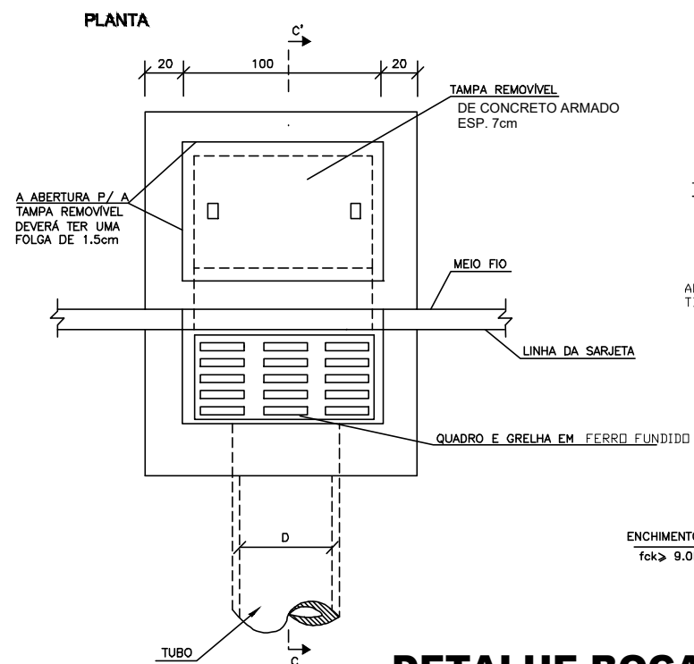
DETALHE BOCA DE LOBO SEM ESCALA
