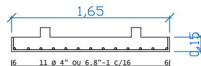
ARMADURA DA LAJE SUPERIOR ARMADURA DA LAJE INFERIOR
