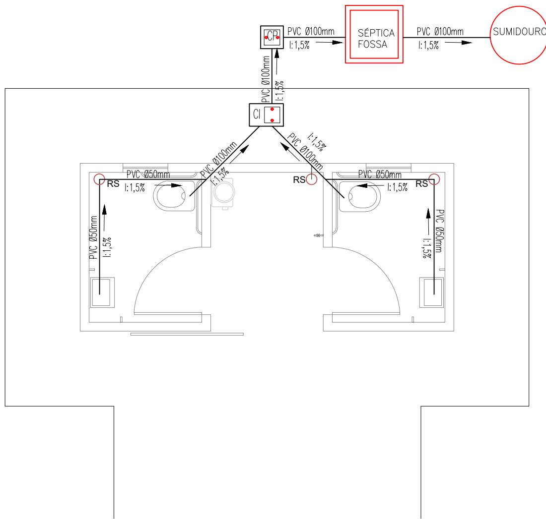
PLANTA BAIXA – ESGOTO SANITÁRIO ESC.1/50
