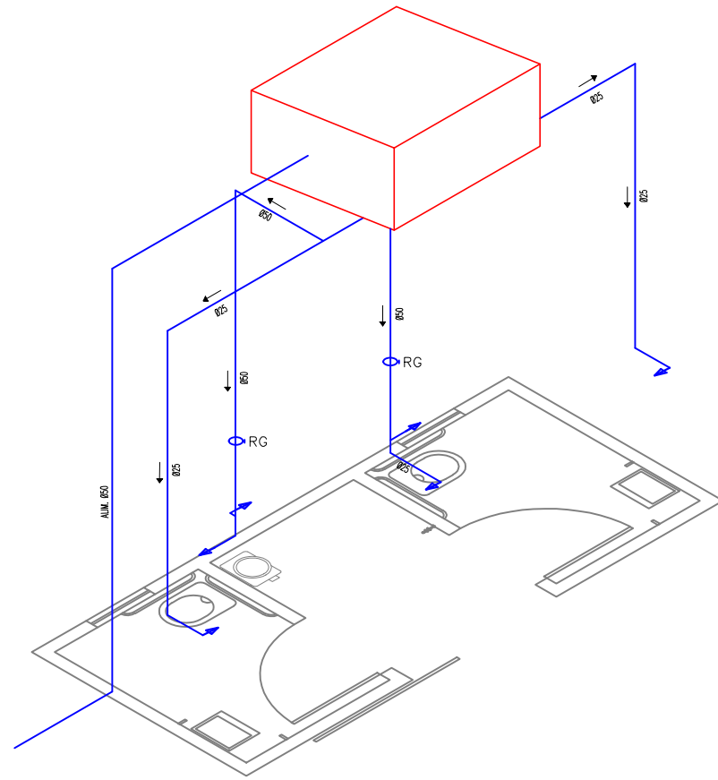
DET. ISOMÉTRICO ÁGUA FRIA ESCALA 1:50
