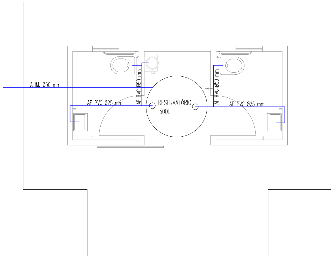
PLANTA BAIXA – ÁGUA FRIA ESC.1/50
