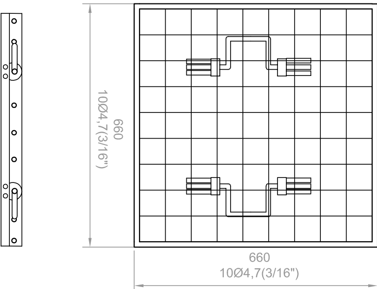
FERRAGEM
