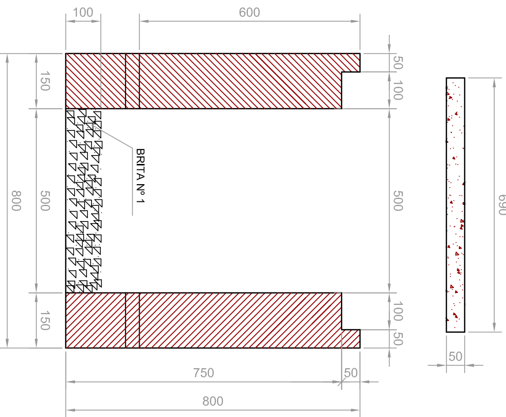
CORTE A-A'
