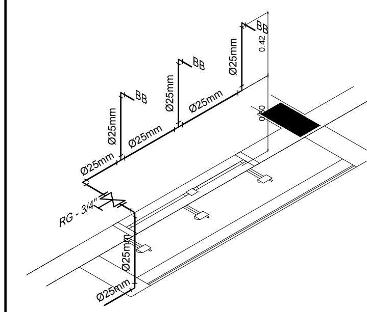
ISOMÉTRICO 1 ESC. 1:25
