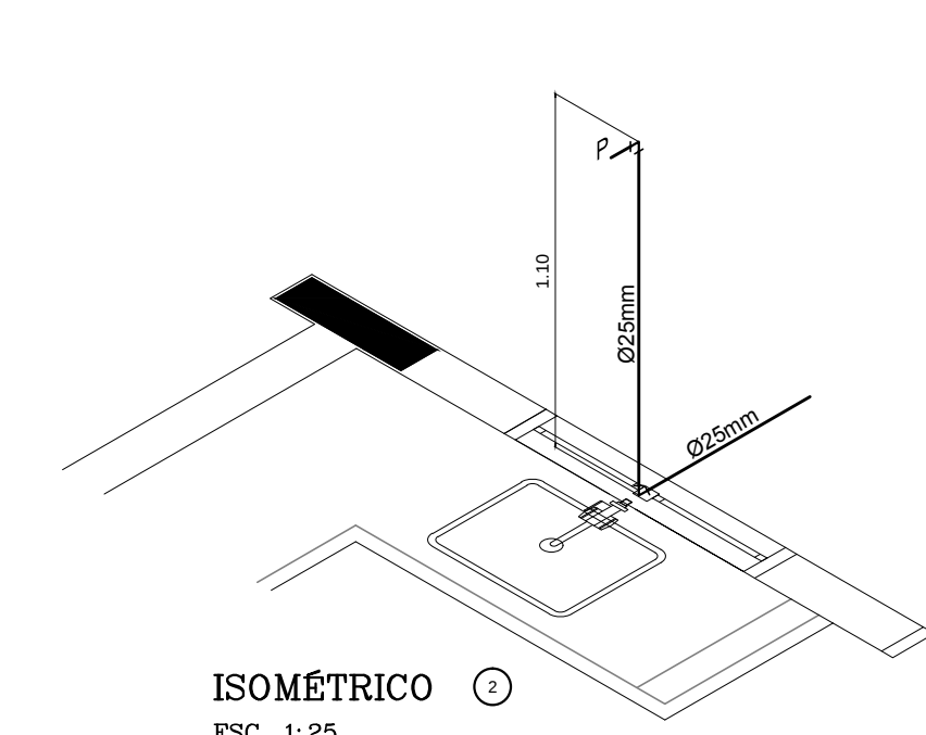
ISOMÉTRICO 2 ESC. 1:25
