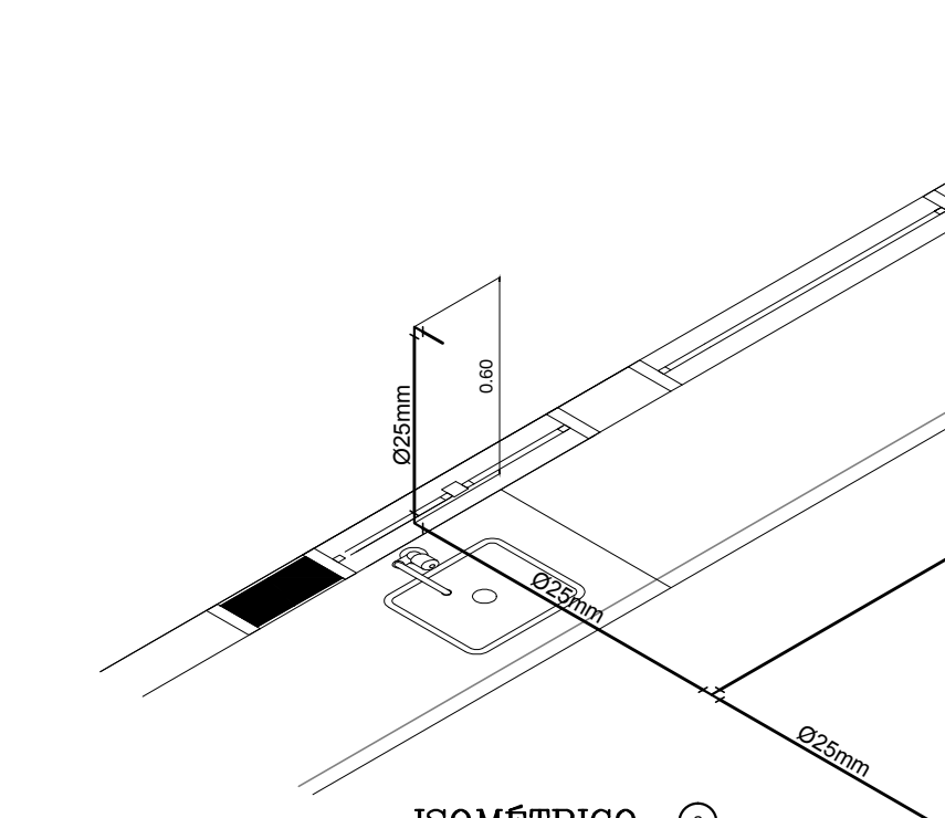
ISOMÉTRICO 4 ESC. 1:25
