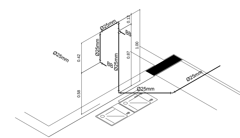
ISOMÉTRICO 6 ESC. 1:25
