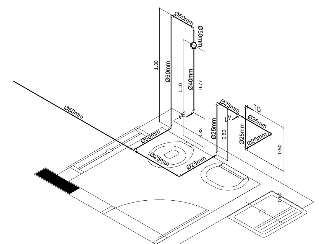
ISOMÉTRICO 7 ESC. 1:25
