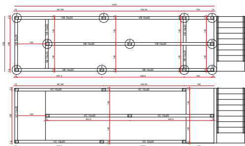
PLANTA ESTRUTURAL - RAMPA 01 ESCALA 1:50
