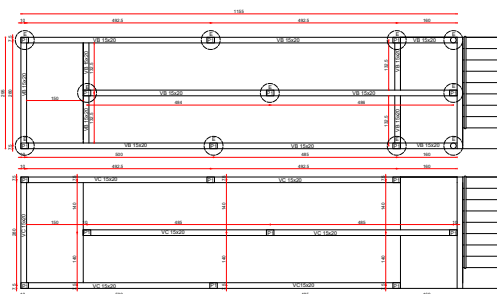
PLANTA ESTRUTURAL - RAMPA 02 ESCALA 1:50
