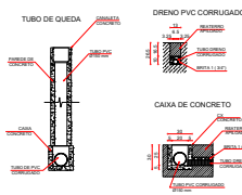
DETALHE DRENAGEM ESCALA 1:25
