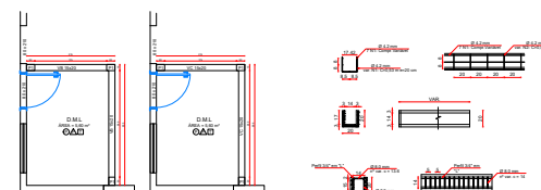
PLANTA ESTRUTURAL D.M.L. ESCALA 1:50
