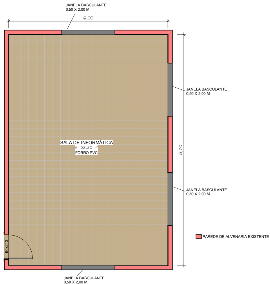
1 TÉRREO 1 : 50
