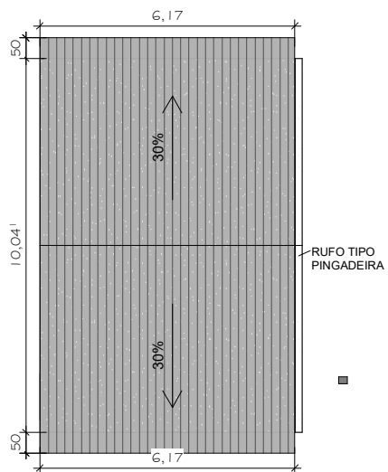
2 PLANTA DE COBERTURA 1 : 100
